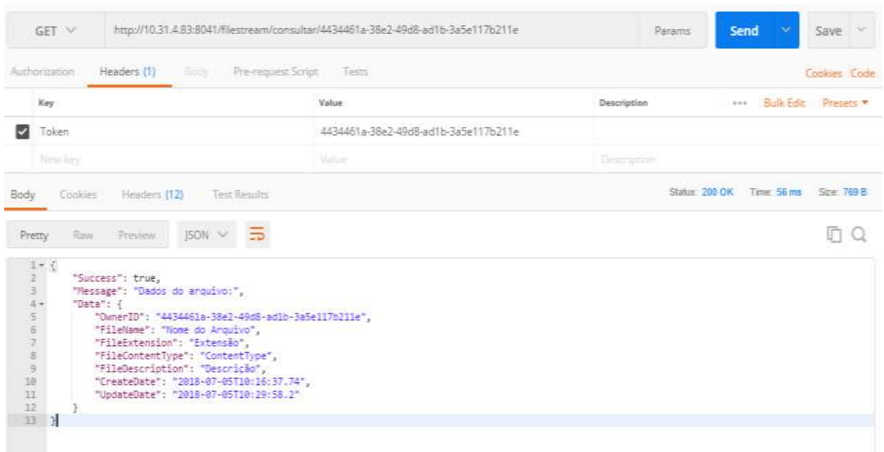
Figura – Consulta de documentos através do Postman
