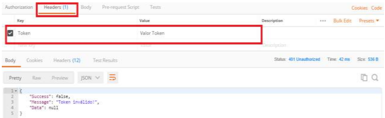
Figura – Passagem do token através do cabeçalho da requisição
