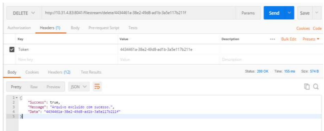
Figura – Exclusão de documentos através do Postman
