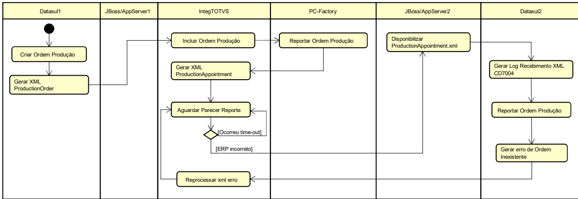
Diagrama Integração TOTVS MES
